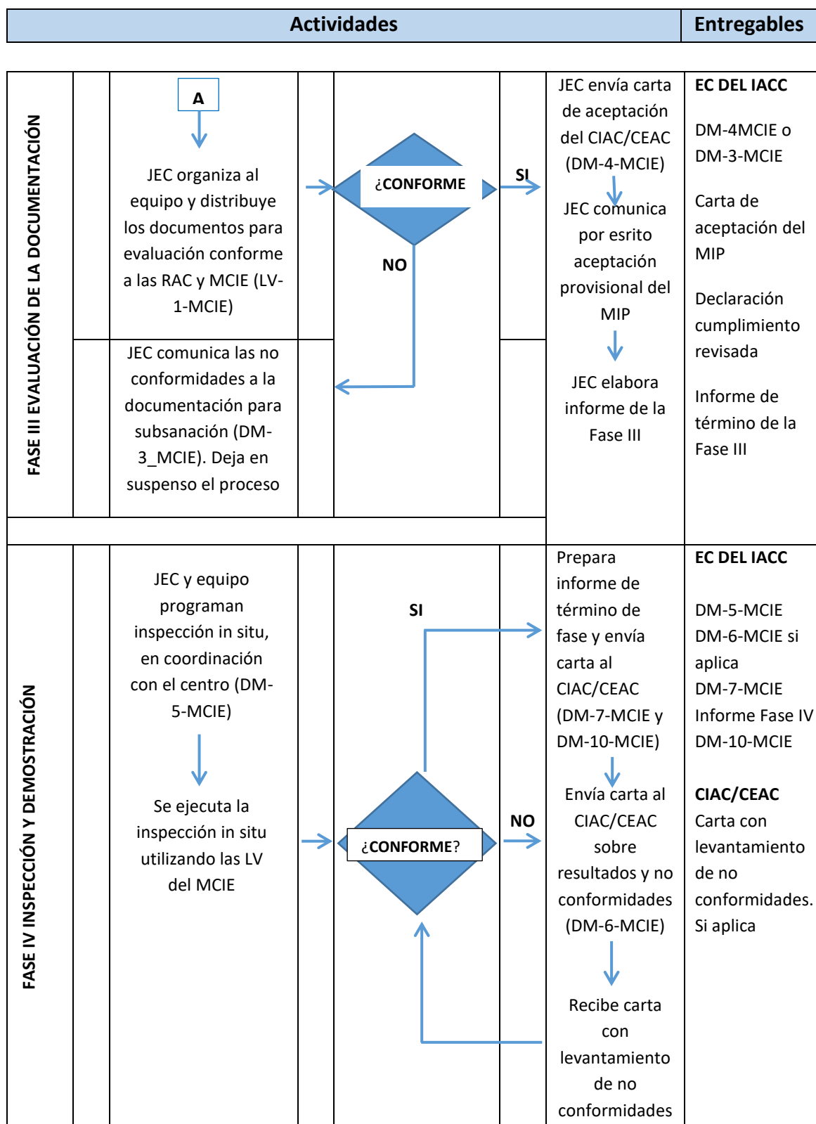
Figura II-2-3 Flujograma del proceso de certificación de un CIAC/CEAC
