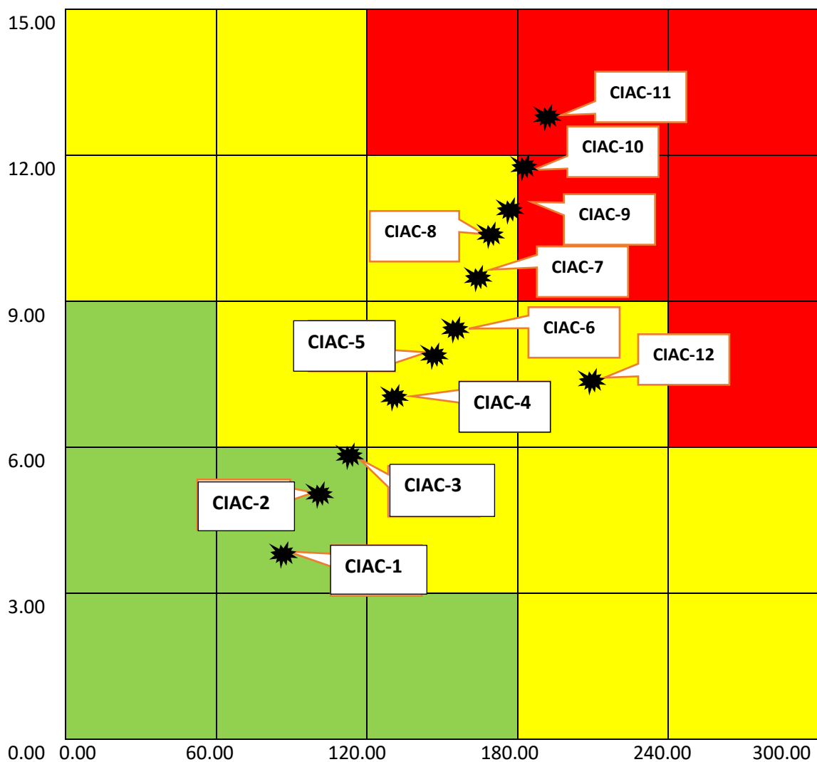
Figura III-3-3 – Priorización de la RBS
